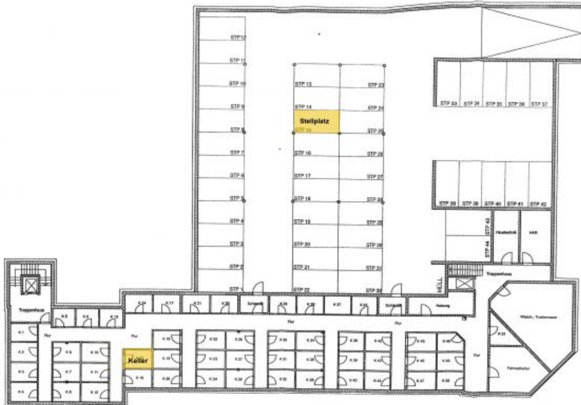
Grundriss Keller / Tiefgarage
