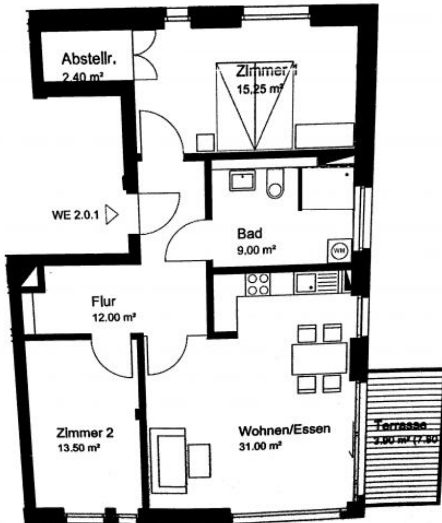
Grundriss Erdgeschoss
